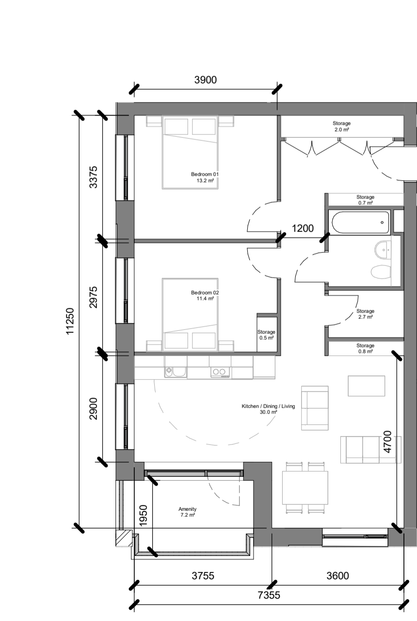
2B4P-Type E1 & E2 (Mirrored) 1: 100
